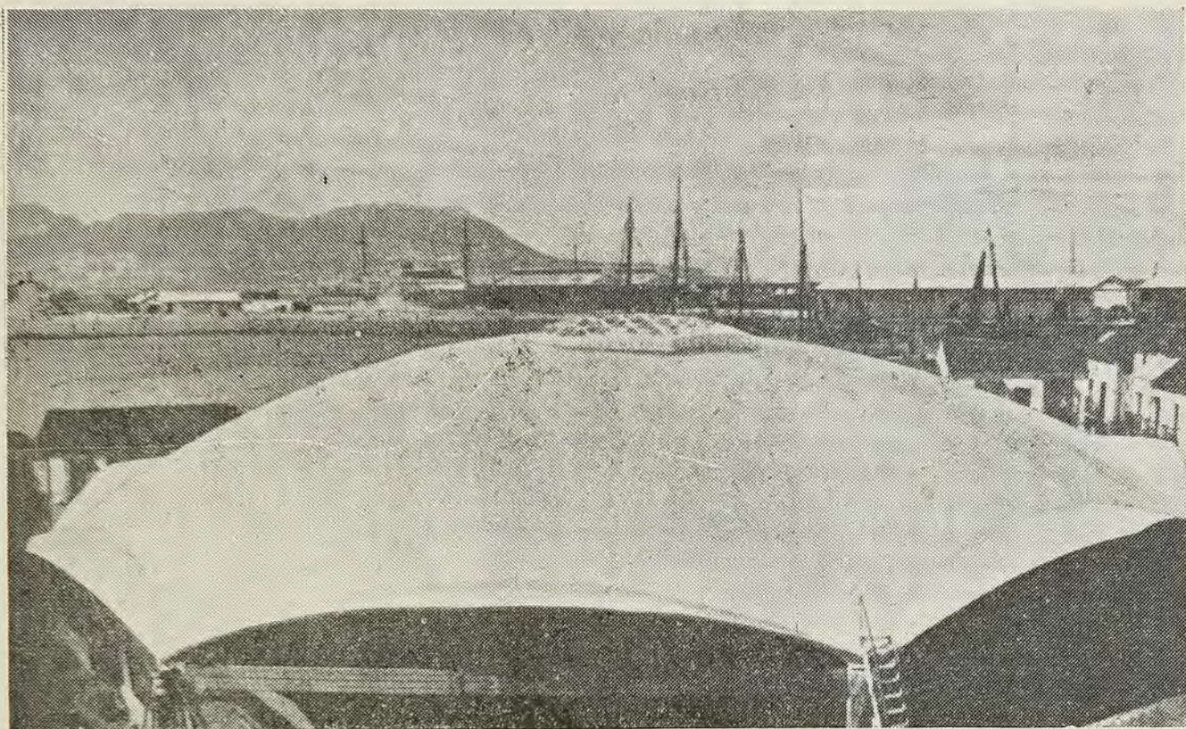
Fig. 9.—Vista exterior del casquete y lucernario.—Obsérvese el aro octogonal con sus barras de fierro tensadas antes de hormigonarse.
