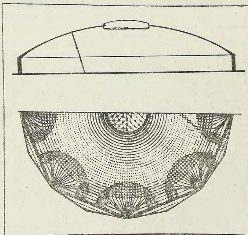
Fig. 8.—Corte y armadura de la bóveda.
